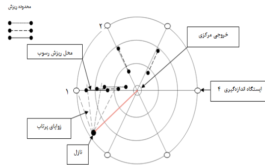
شکل ۲: موقعیت پرتاب جت آب در مخزن
