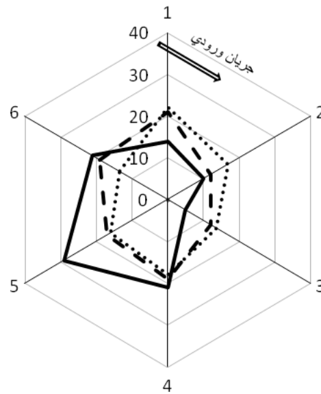
شکل ۵: الگوی کمی رسوب گذاری با ریزش رسوب در قسمت بینابینی شعاع مخزن در ایستگاه‌های ۱، ۲ و ۳ Figure 5: Quantity pattern of sedimentation in station 1, 2 and 3 in middle position
