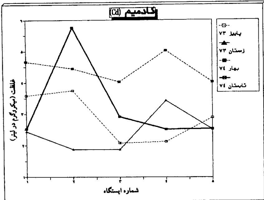
شکل ۴: مقایسه میزان کادمیم در آب ایستگاههای مورد مطالعه در فصول مختلف
