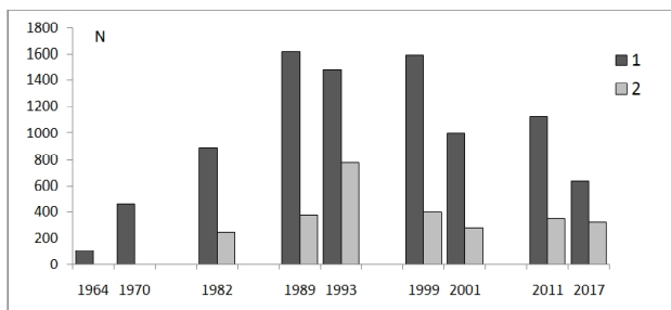
Рис. 2. Многолетнее изменение численности летнего зоопланктона ( N , тыс. экз./ m^3 ) в вершинной (1) и в центральной (2) части залива
