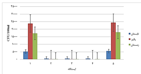
شکل ۵: مقایسه تغییرات میانگین کلی فرم کل در ایستگاه‌های مورد مطالعه سد سیمره در فصول مختلف
