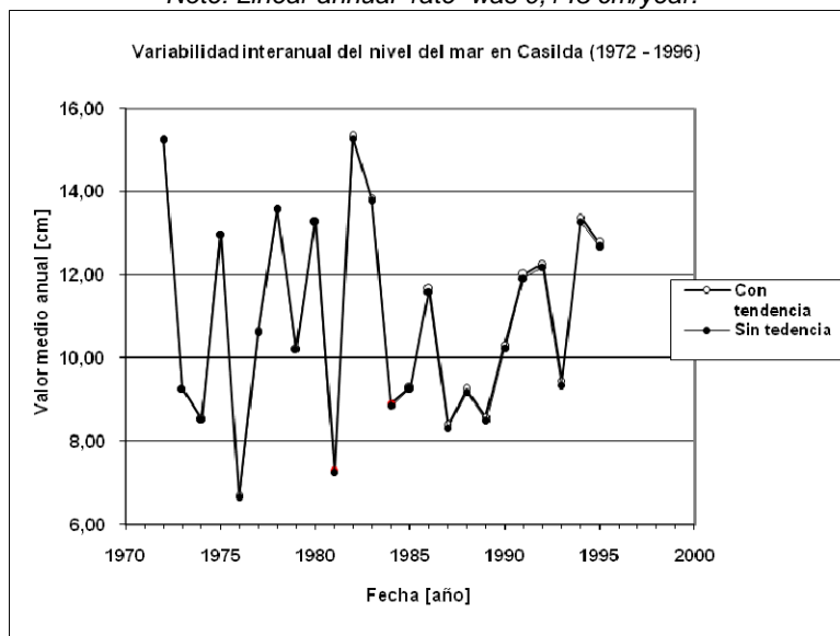
Figura 6. Variabilidad interanual del nivel del mar en Casilda (1972 – 1995).
