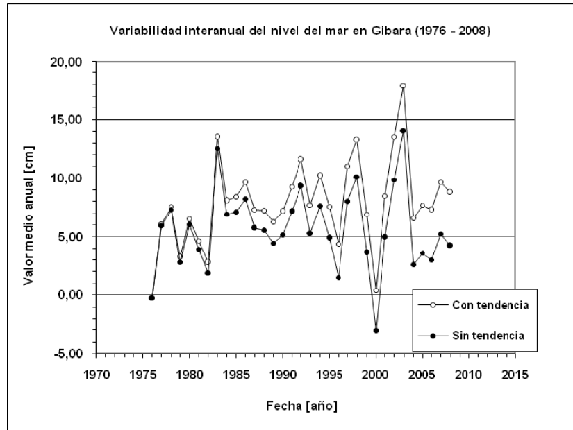
Figura 5. Variabilidad interanual del nivel del mar en Gibara (1976 – 2008).
