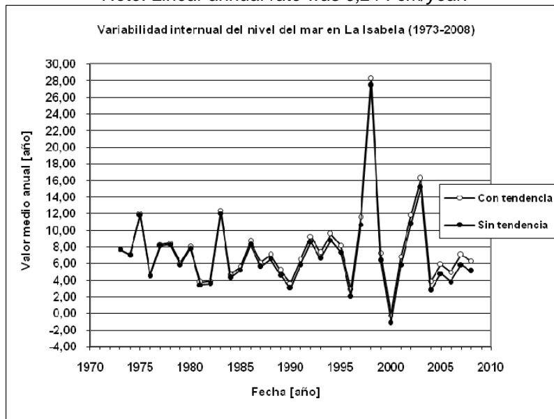
Figura 4. Variabilidad interanual del nivel del mar en La Isabela (1973 – 2008).
