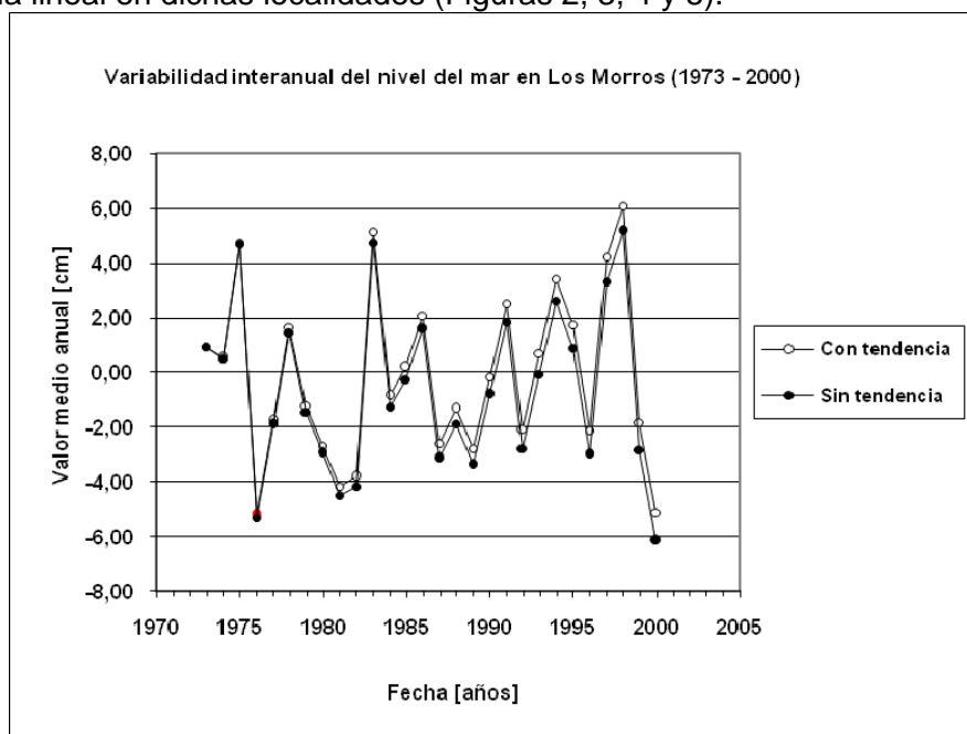
Figura 2. Variabilidad interanual del nivel del mar en Los Morros (1973 – 2000).
