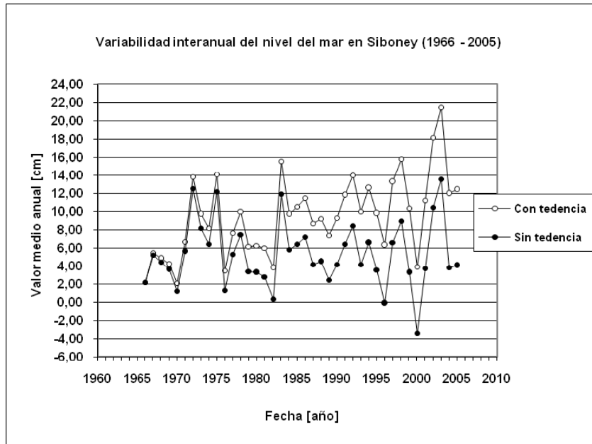
Figura 3. Variabilidad interanual del nivel del mar en Siboney (1966 – 2005).
