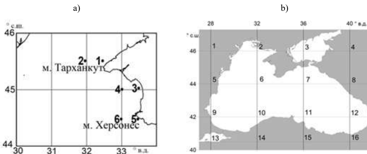
Рис. 1. Точки оцифровки карт спутниковой альтиметрии в районе промысла шпрота у западных берегов Крыма (а) и сетка мониторинга приземного поля атмосферного давления над Азово-Черноморским регионом (б)
