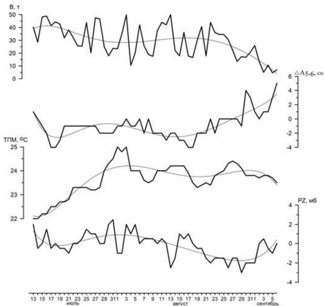
Рис. 2. Изменения средней промысловой нагрузки ( B , т), показателя характера прибрежных течений ( \Delta A_{5-6} ), средней ТПМ в районе промысла ( ^{\circ}\text{C} ) и показателя атмосферной циркуляции PZ (сглажены полиномиальной функцией 6-й степени)
