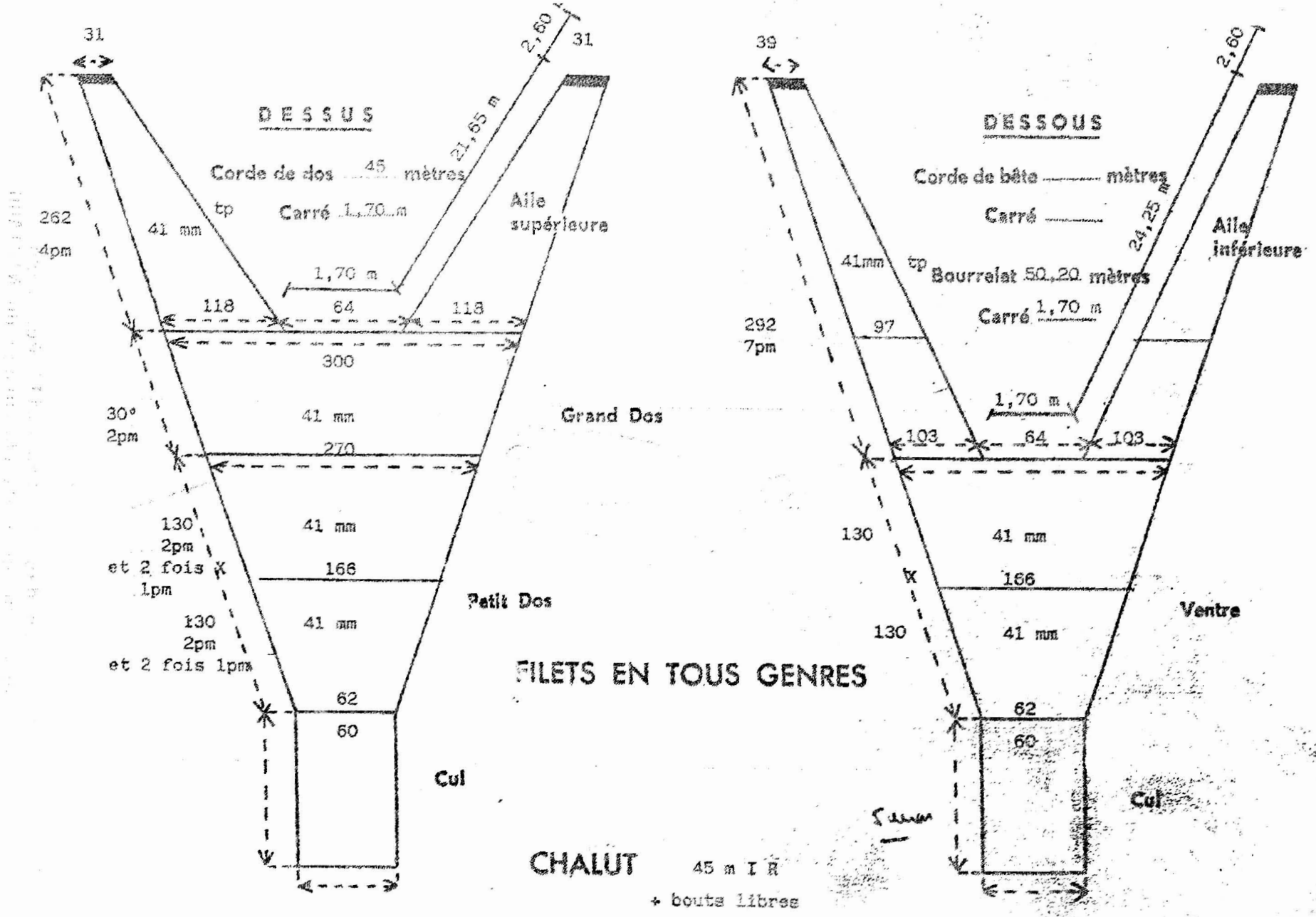
Annexe n° 1: plan du chalut irlandais utilisé durant les campagnes de chalutage du N/O N°DIAGO.
