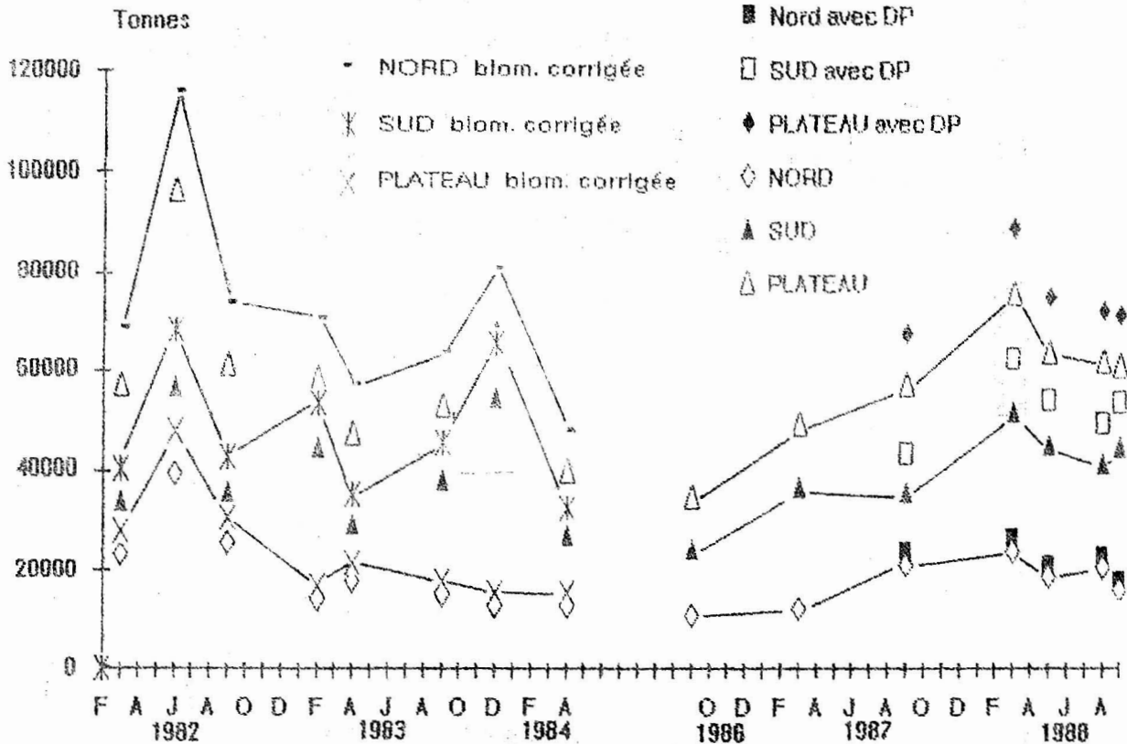
Figure n° 24: Biomasse démersale apparente (et corrigée) du plateau continental mauritanien, évaluée par les campagnes du N/O N'DIAGO, de 1982 à 1988.
