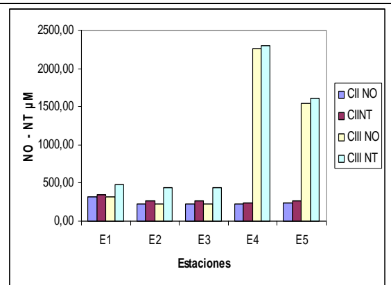
Figura 5. Distribución del nitrógeno orgánico NO y nitrógeno total NT en la laguna (I: febrero/2006, II: mayo/2007 y III: octubre/2007).
