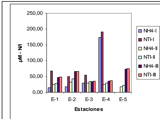
Figura 4 Distribución del amonio NH_4 y del nitrógeno total inorgánico NTI en la laguna (I: febrero/2006, II: mayo/2007 y III: octubre/2007).
