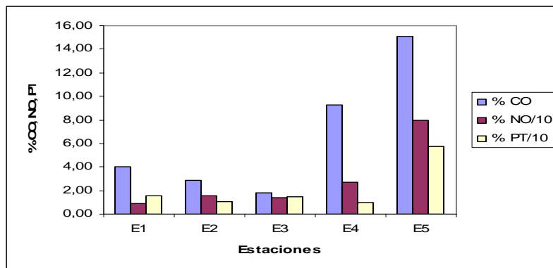
Figura 7 Concentraciones carbón orgánico CO, nitrógeno orgánico NO y fósforo total PT en sedimentos superficiales en la laguna El Doctor.
