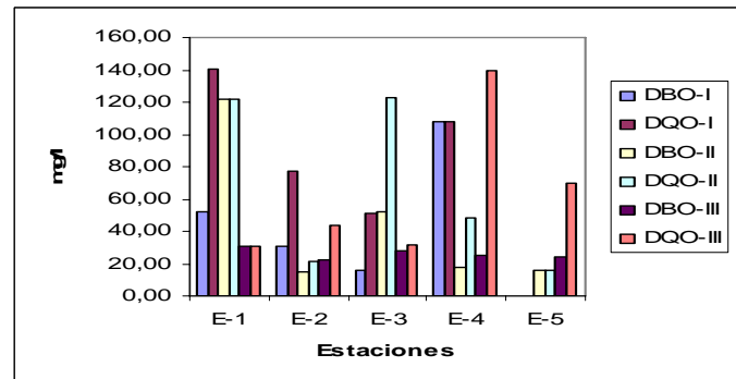
Figura 3 Distribución de la DBO 5 y DQO en la laguna (I: febrero/2006, II: mayo/2007, III: octubre/2007).
