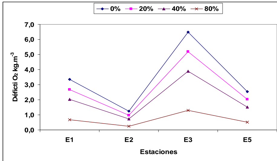
Figura 8. Déficit de oxígeno disuelto estimado a partir de los diferentes porcentajes de reducción de los residuales sin tratamiento (0 %) y tratamiento de 20%, 40% y 80 % correspondiente a mayo del 2007.
