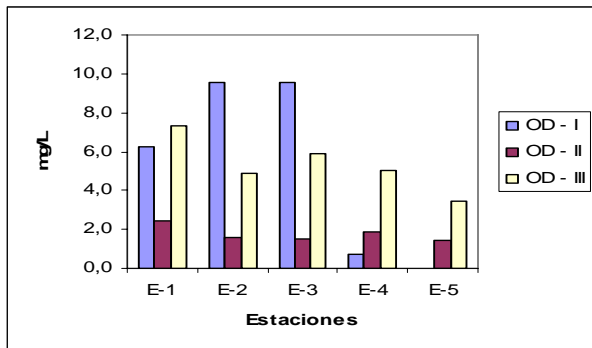
Figura 2. Distribución del oxígeno disuelto OD en la laguna (I: febrero/2006, II: mayo/2007, III: octubre/2007).
